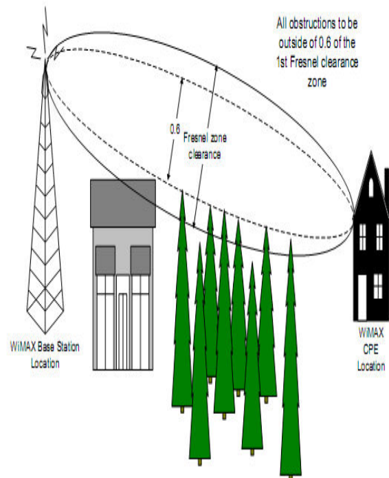
Figure.1. LOS Fresnel zone
